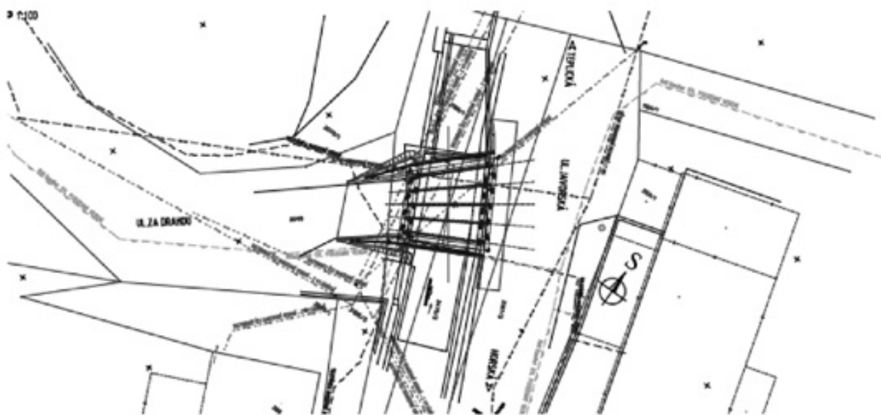
Celková koordináční situace stavby Rekonstrukce mostu 29b-01 v ulici Za Drahou
